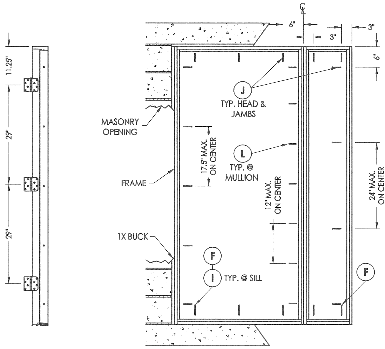
HINGE JAMB
